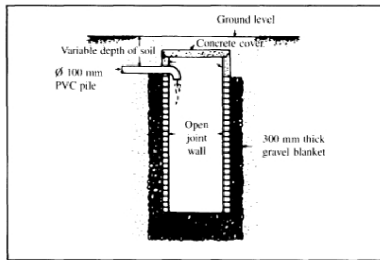
Figure 56 : SIMPLE SOAKAWAY
